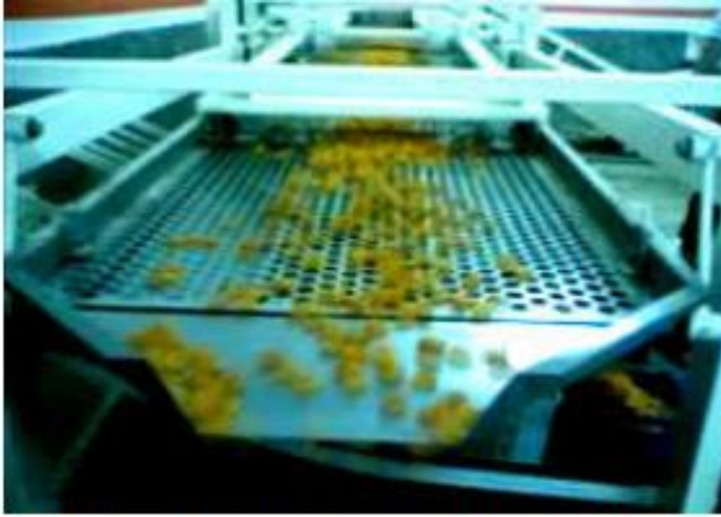
Resim 2.5: Düz elek tipi sınıflandırma sistemi
