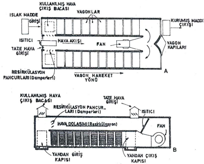
Zıt Akış Tünel Kurutucu
